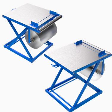
Mesa de elevación con portarodillo
